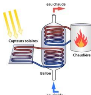
Appoint séparé : chaudière
